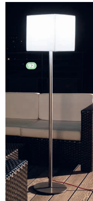
92 CUBICO Lampe. Polyéthylène anti-UV, antigel. 230 V - 50 Hz. Livrée sans ampoule. Alimentation secteur. IP55. Piètement en métal et peinture époxy. Câble rouge de 3 m. Coloris : blanc. Design Italien. L30 X H155 X P30 cm.
