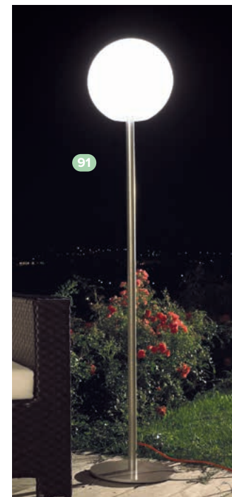
90 BIANCA Lampe d'intérieur et d'extérieur. Polyéthylène anti-UV, antigel. 230 V - 50 Hz. Livrée sans ampoule. Alimentation secteur. IP55. Piètement en métal et peinture époxy. Câble rouge de 3 m. Coloris : blanc. Design Italien. Ø30 X H165 cm. 91 RONDO Lampe. Polyéthylène anti-UV, antigel. 230 V - 50 Hz. Livrée sans ampoule. Alimentation secteur. IP55. Piètement en métal et peinture époxy. Câble rouge de 3 m. Coloris : blanc. Design Italien. Ø30 X H165 cm.
